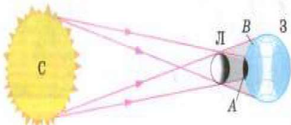
Рис. 4. Солнечное затмение.
