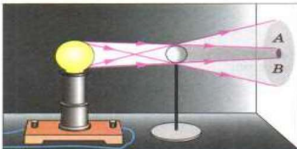
Рис. 2. Получение полутени.
